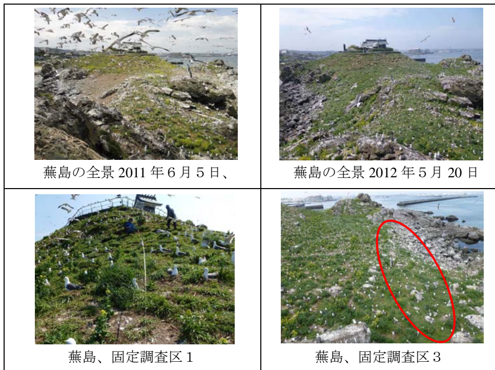
図 2.6 燕島（青森県八戸市）の海鳥繁殖地位置図と景観写真
