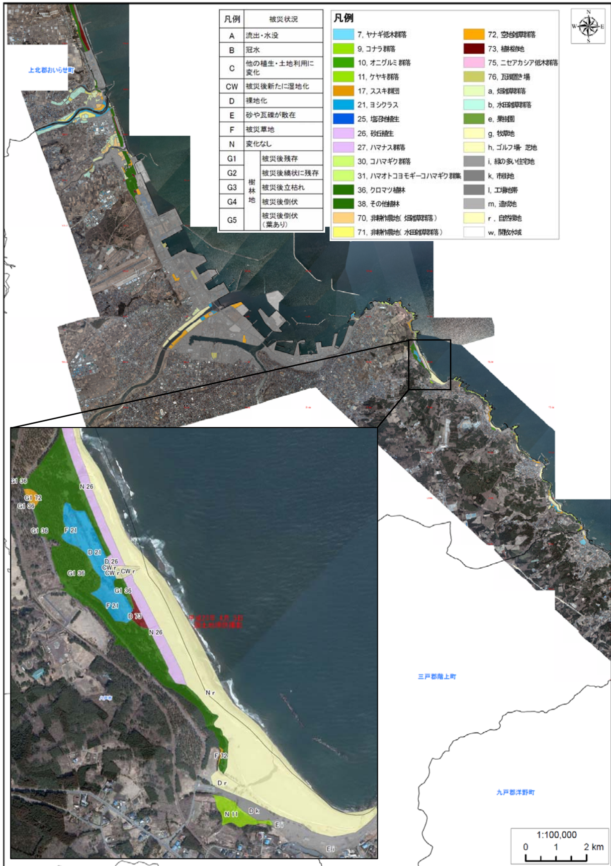
図 2.4 震災後植生図（八戸市）
