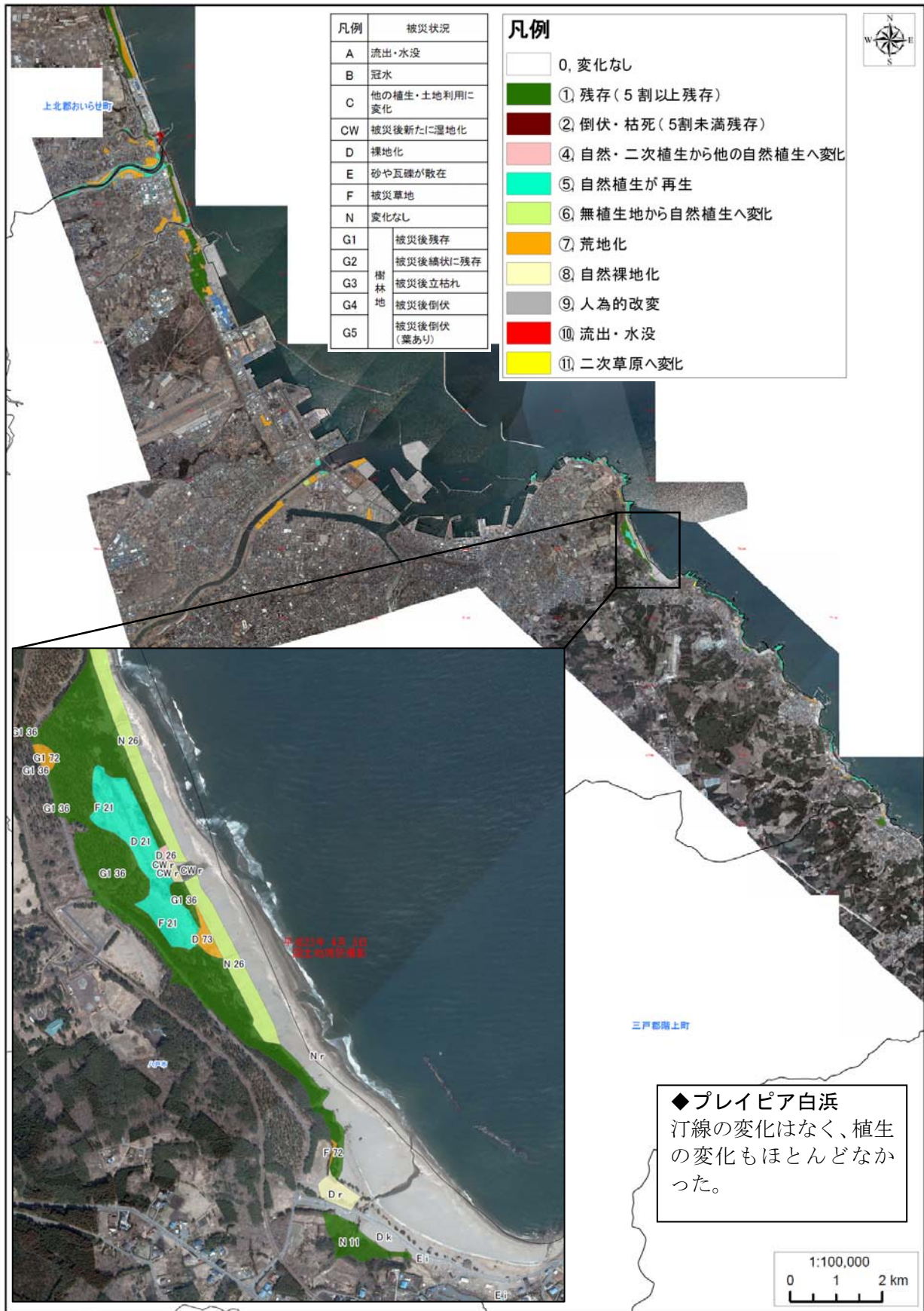
図 2.5 植生改変図 (八戸市)
