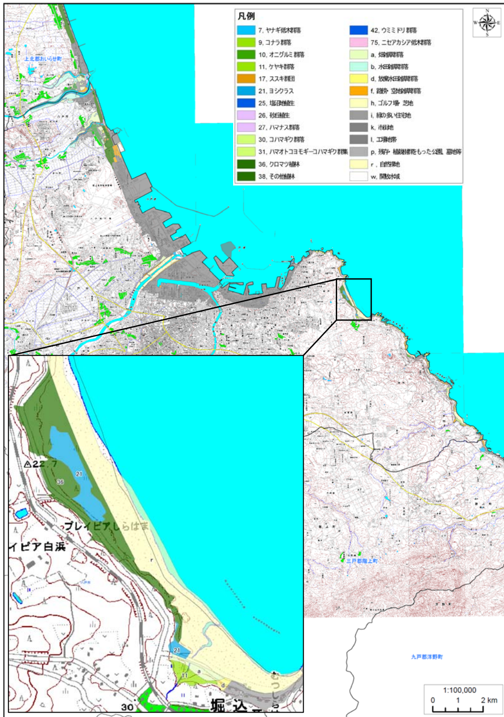
図 2.3 震災前植生図（八戸市）
