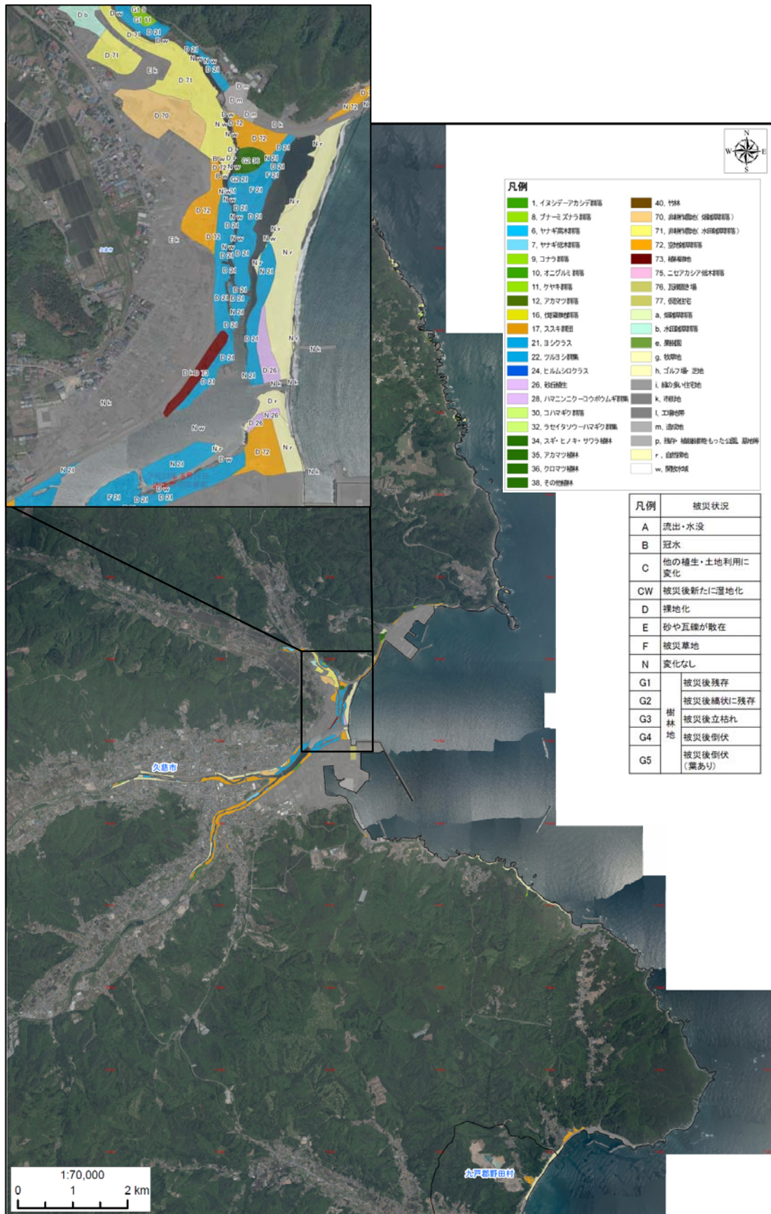
図 2.4 震災後植生図 (久慈市)
