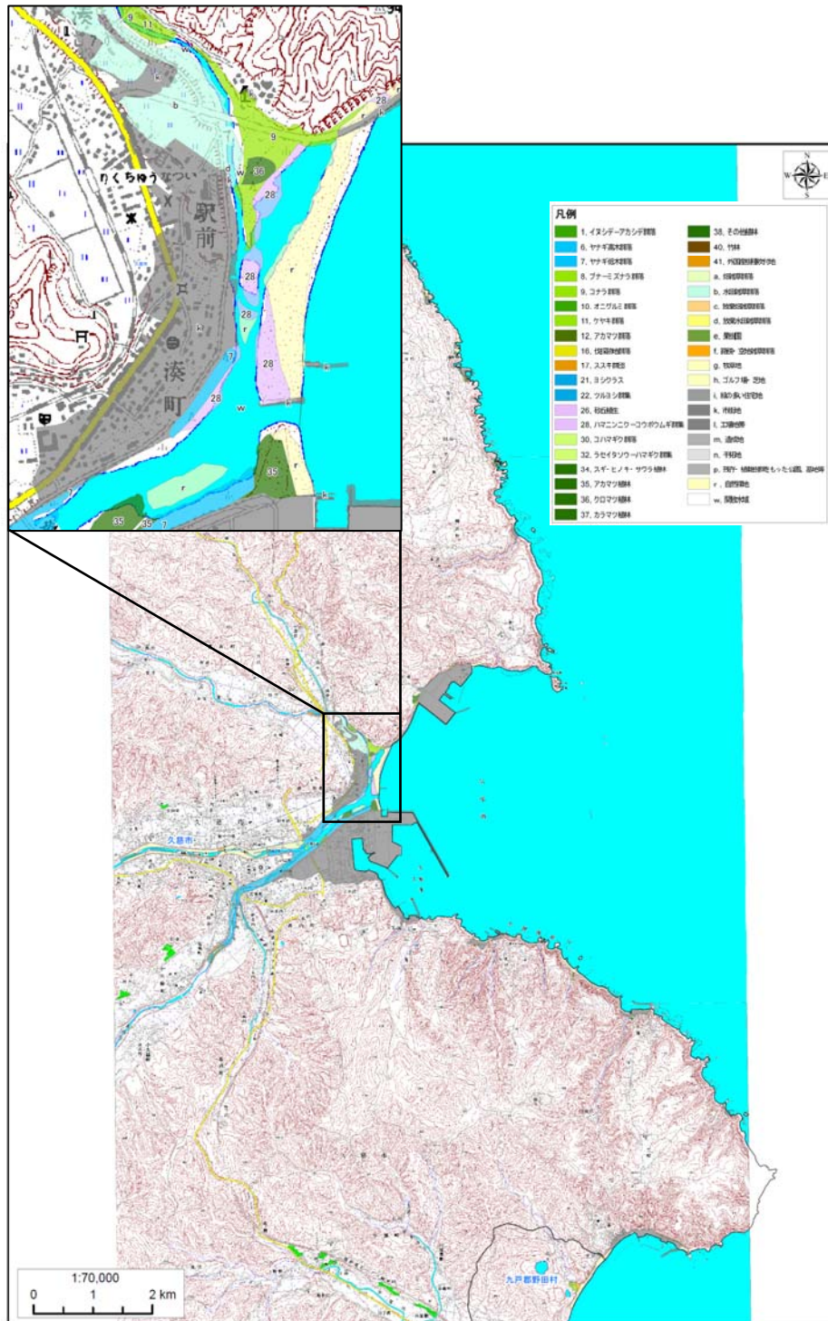
図 2.3 震災前植生図 (久慈市)
