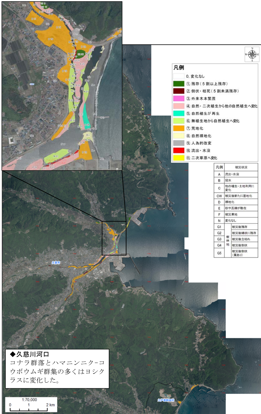
図 2.5 植生改変図 (久慈市)
