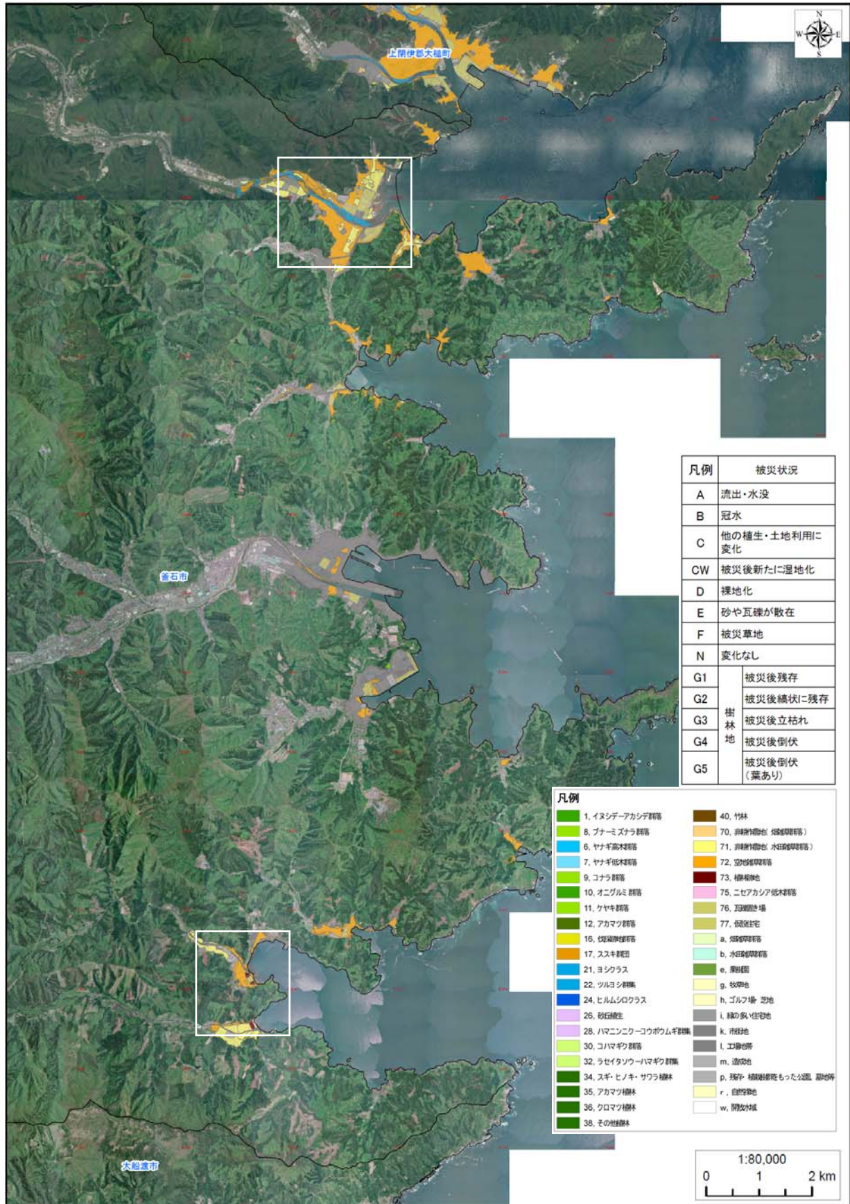
図 2.5 震災後植生図（釜石市）
