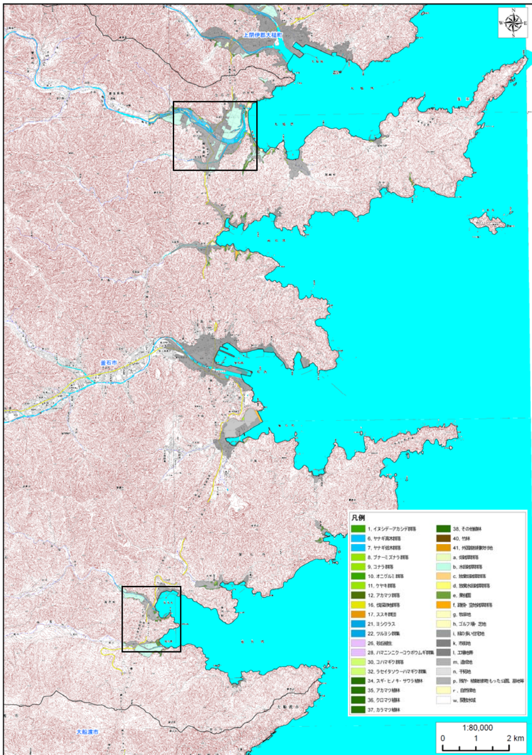
図 2.3 震災前植生図（釜石市）
