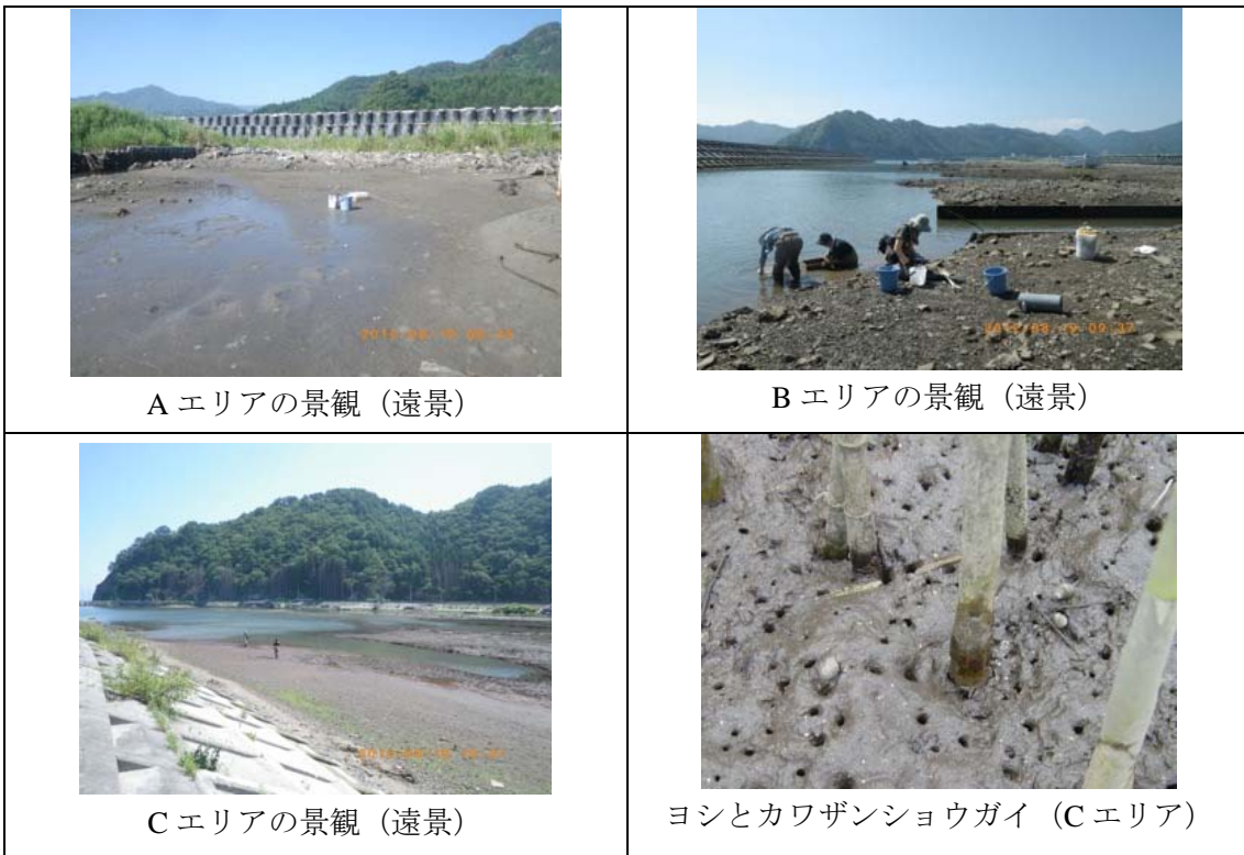
図 2.9 鶺住居川の干潟調査位置と景観写真
