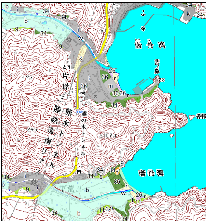
図 2.4 拡大図：震災前植生図（釜石市）
