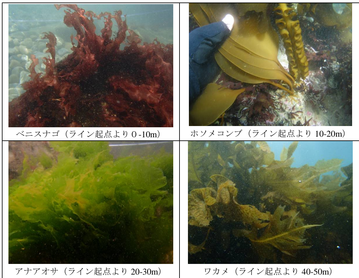
図 2.8 女川湾の藻場調査位置と景観写真
