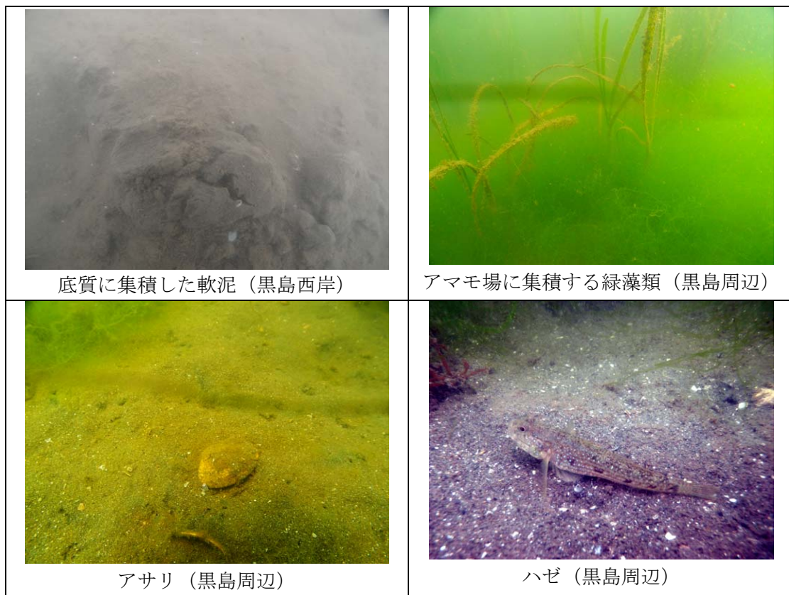
図 2.6 万石浦のアマモ調査位置と景観写真
