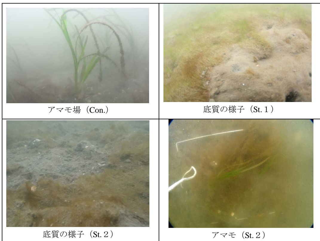
図 2.6 松島湾（寒風沢島）のアマモ場調査位置と景観写真
