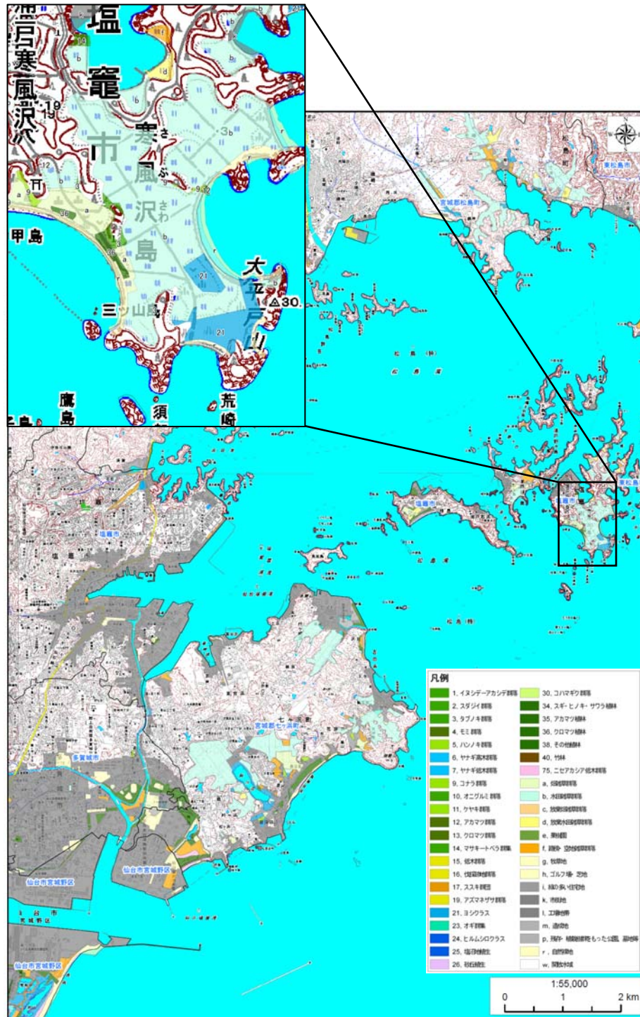
図 2.3 震災前植生図 (塩竈市)
