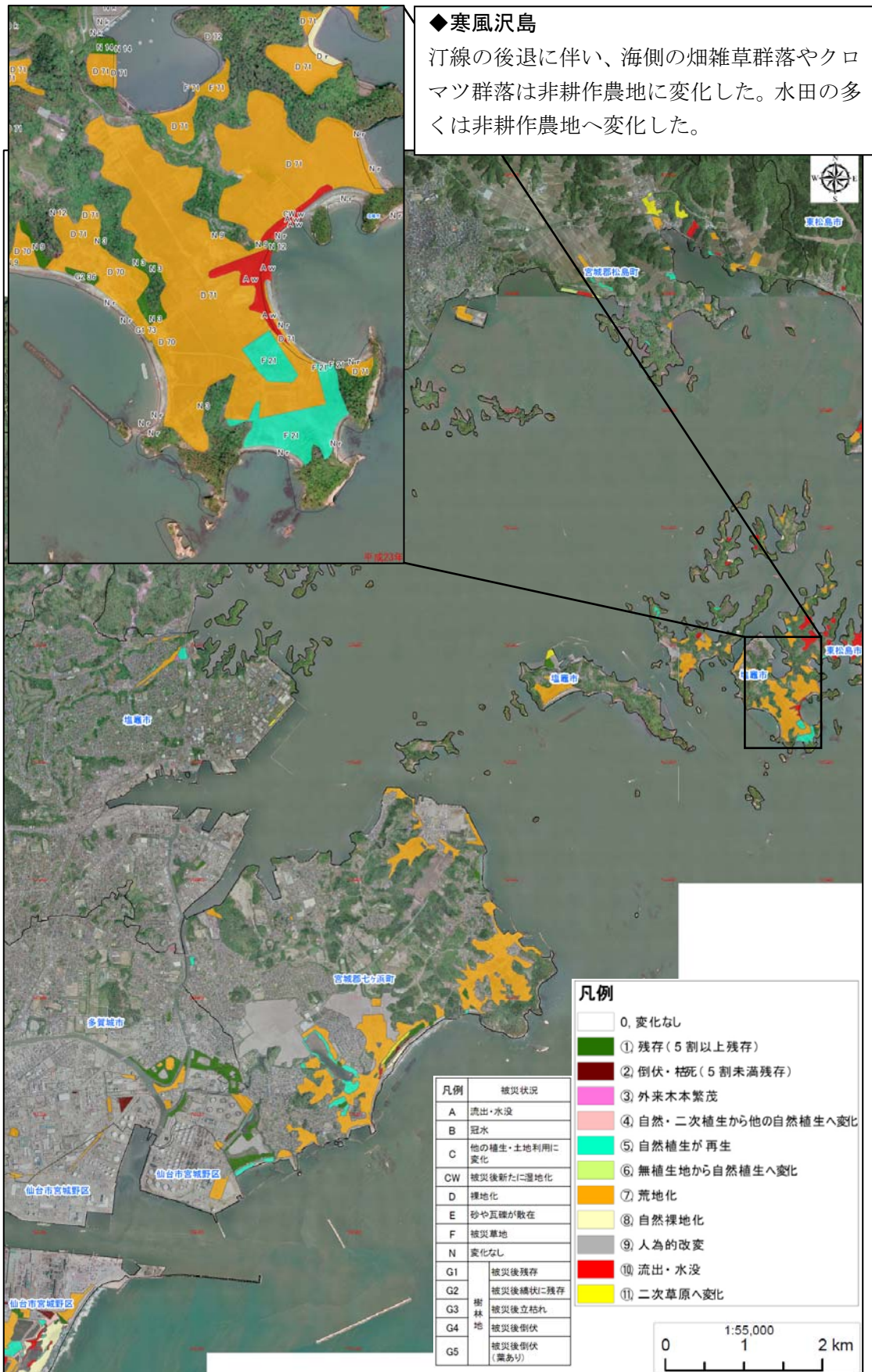
図 2.5 植生改変図(塩竈市)
