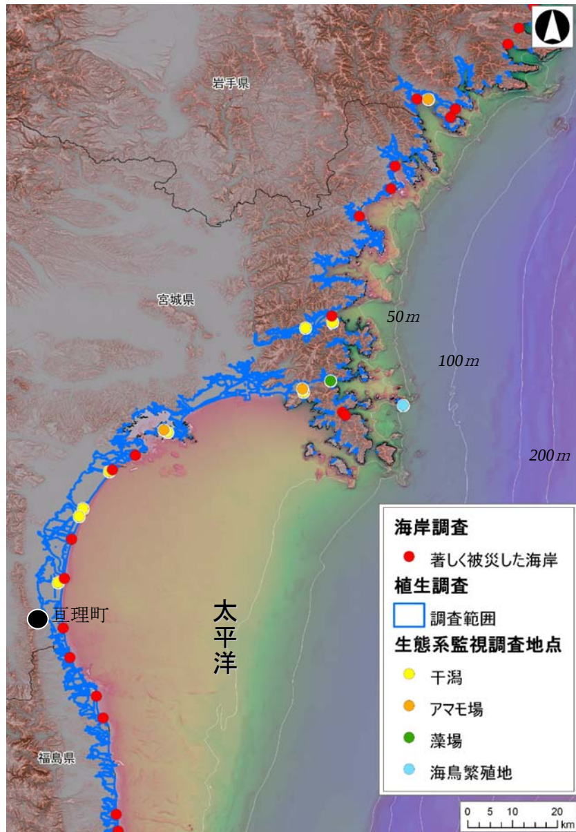
図 2.1 宮城県周辺の海域から陸域の地形
