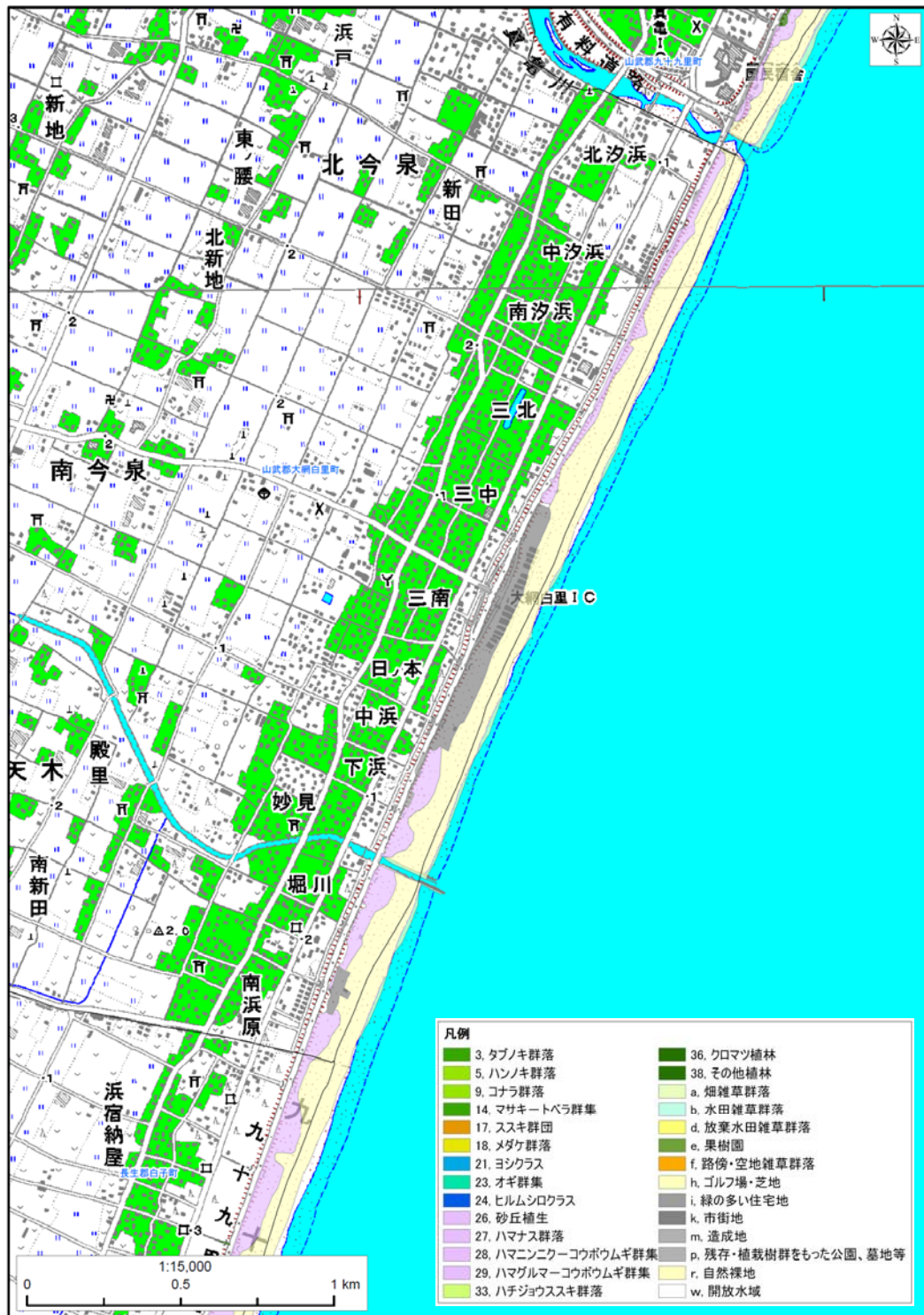
図 2.3 震災前植生図 (大網白里市)
