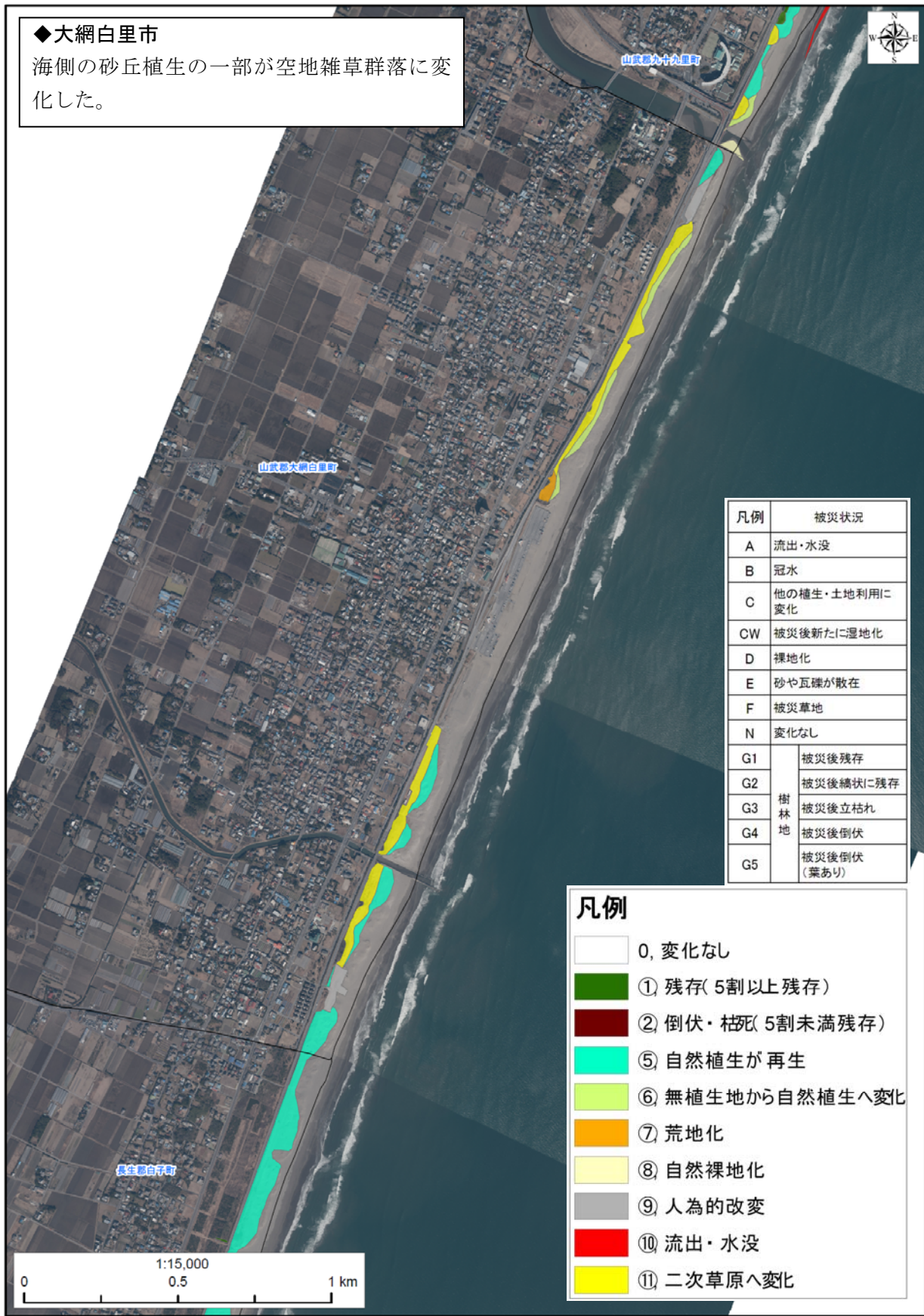
図 2.5 植生改変図 (大網白里市)
