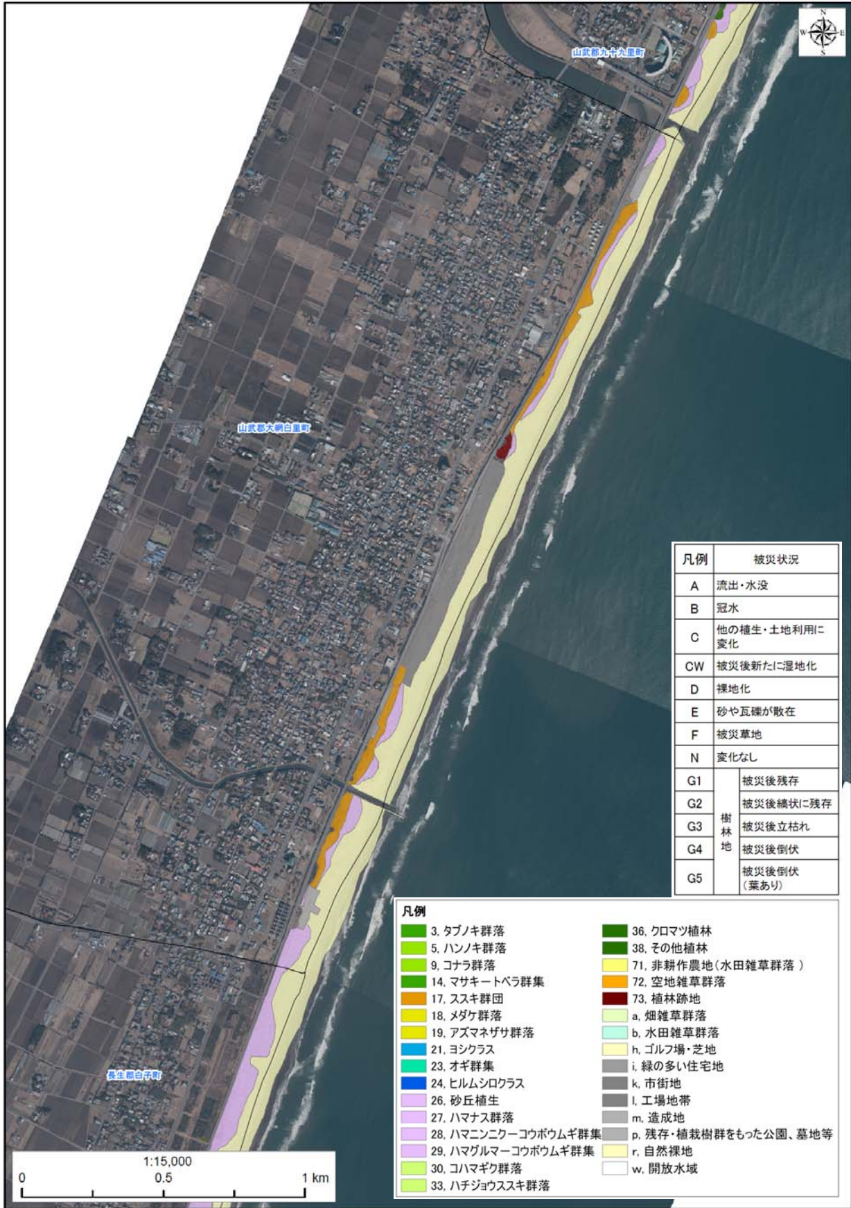
図 2.4 震災後植生図 (大網白里市)
