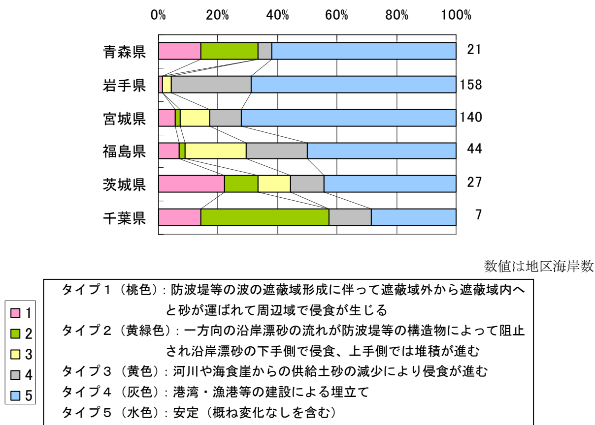
図4.19 県別の海岸の変化要因 (1970 年代－2000 年代)
