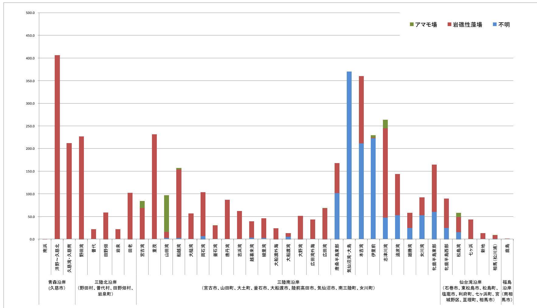
図 6.22 海岸区分別藻場・アマモ場面積
