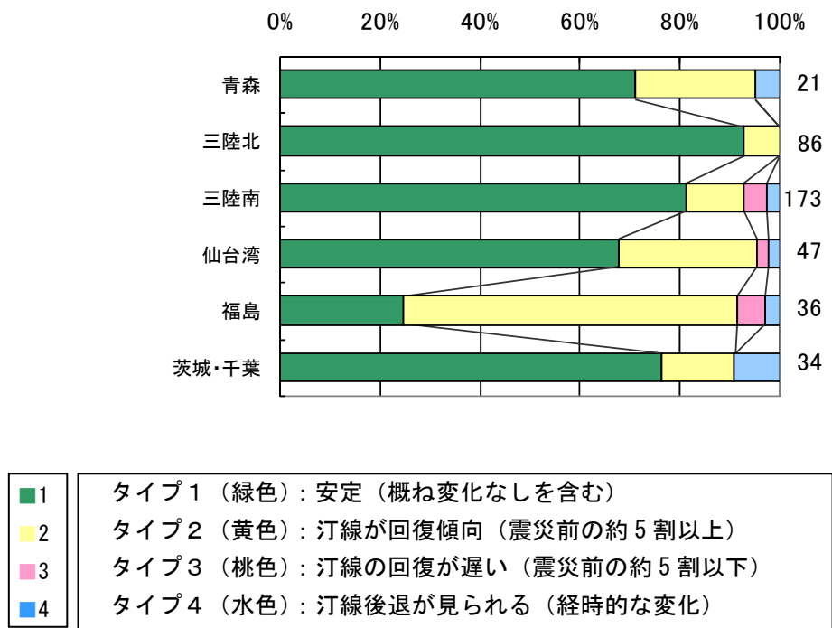
図4.25 県別の海岸の変化状況 (2011 年-2014 年)
