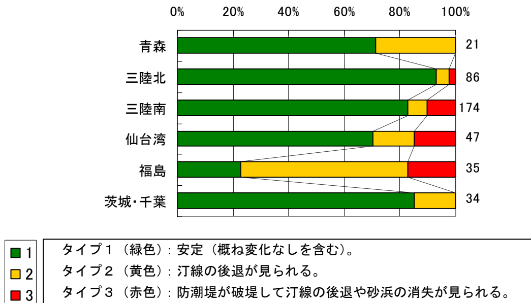
図4.24 沿岸別の海岸の変化状況 (震災後)
