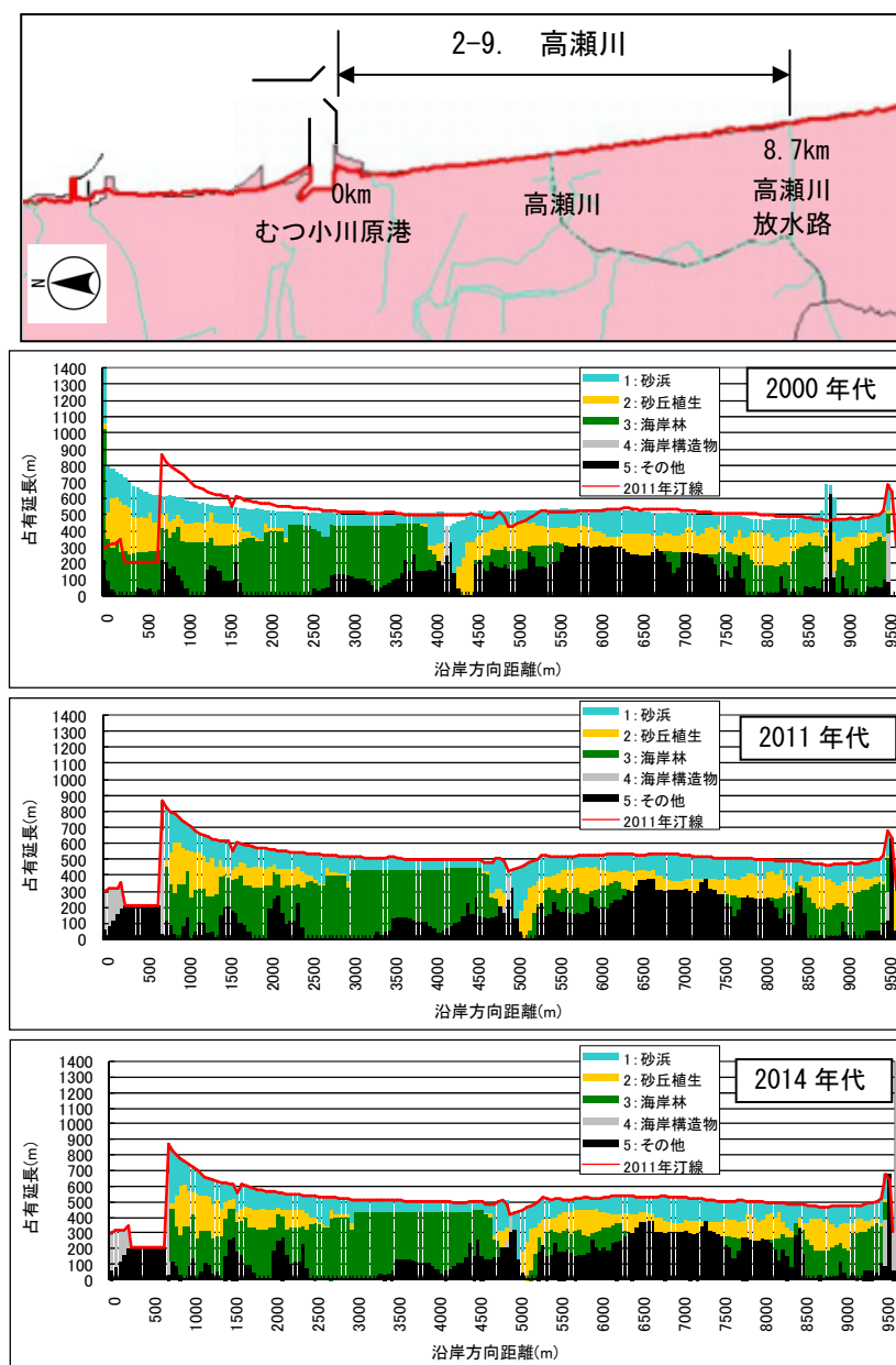
図4.40 六ヶ所村高瀬川
