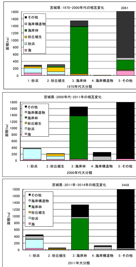
図4.34 土地被覆面積変化の相互関係（宮城県）
