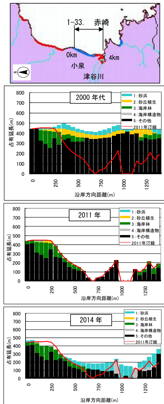
図4.56 気仙沼市赤崎
