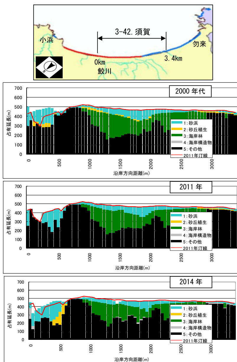
図4.74 いわき市須賀
