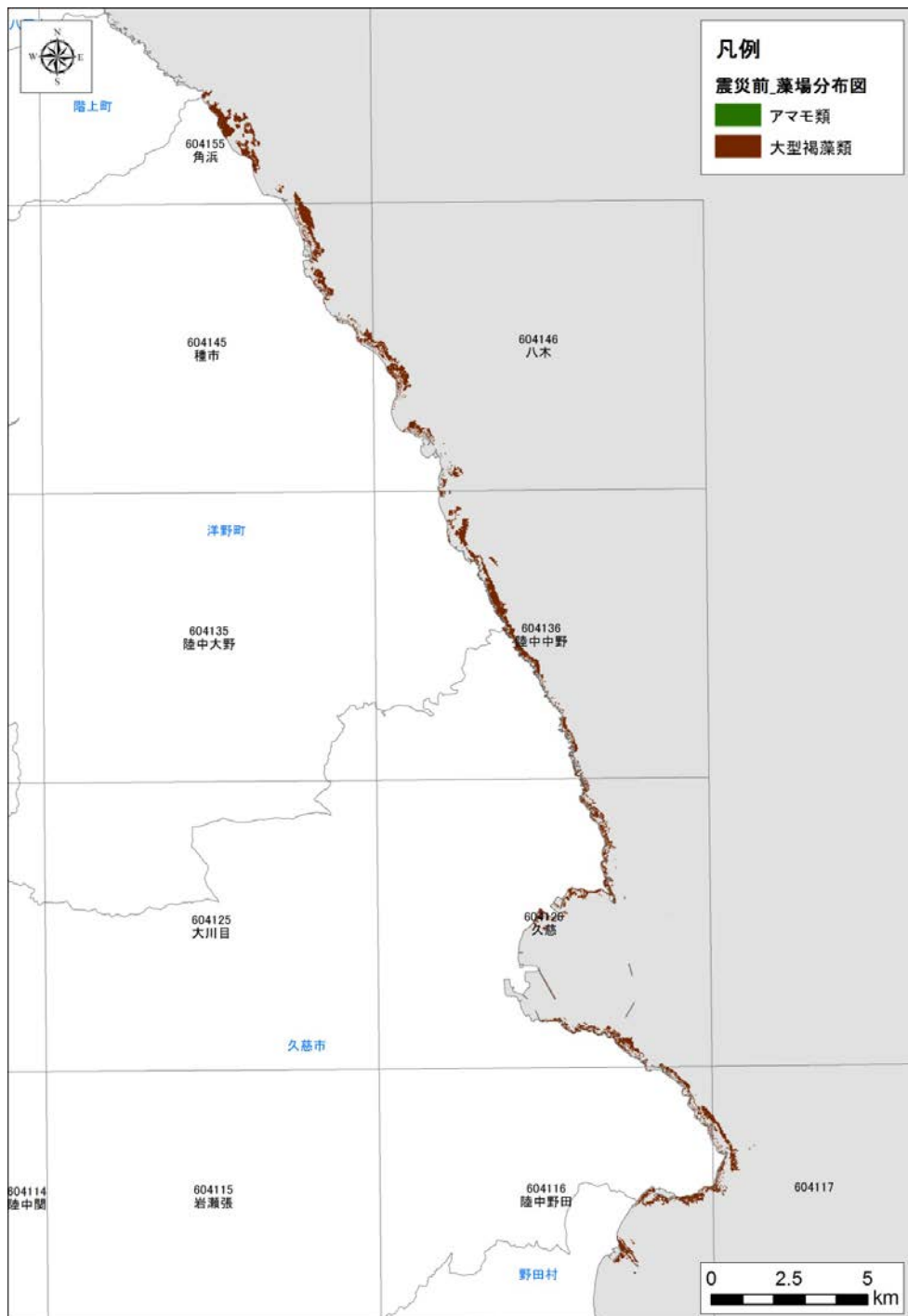
図 2.12 藻場・アマモ場の震災前分布図 (岩手県北部)
