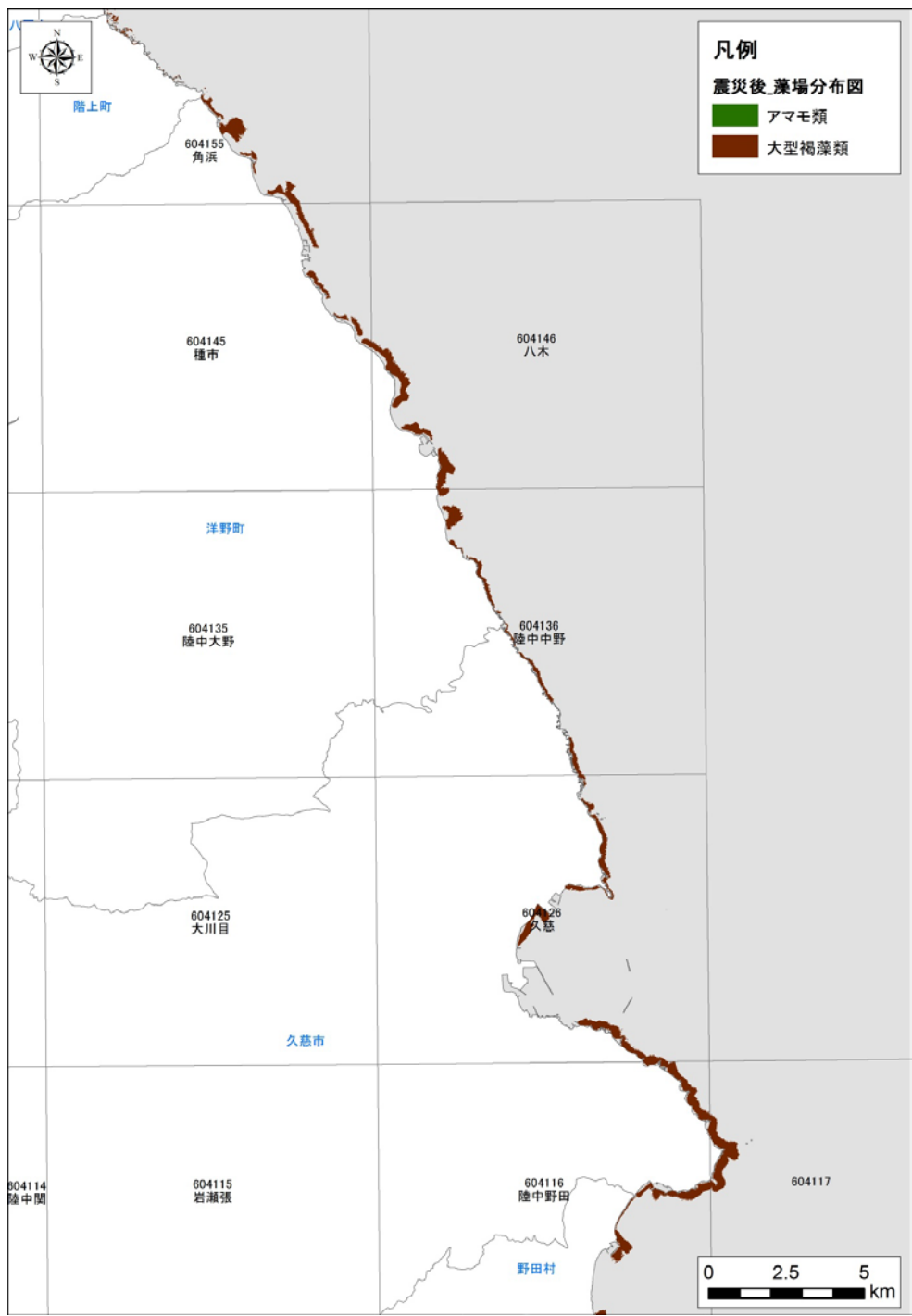
図 2.13 藻場・アマモ場の震災後分布図 (岩手県北部)
