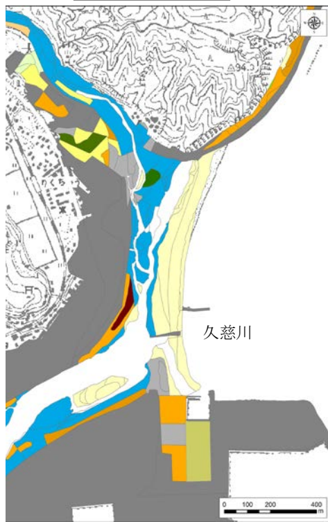
図 2.2 4ヶ年植生図(久慈市)
