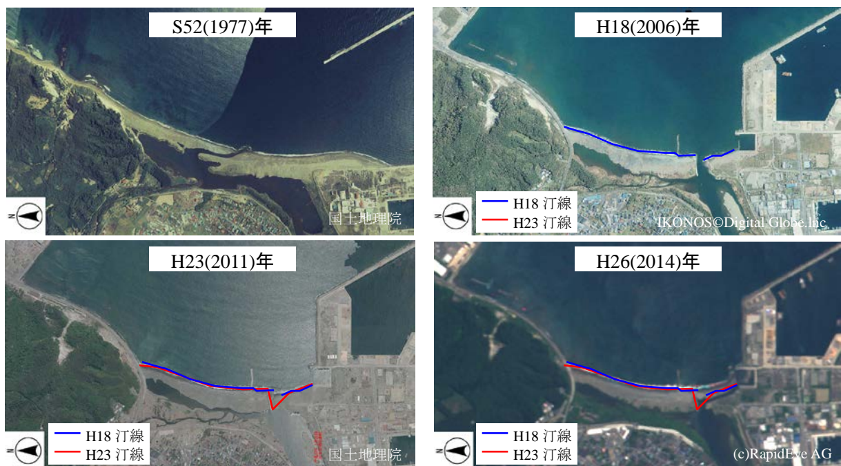
図 2.8 空中写真・衛星画像による海岸の変遷（久慈市久慈川海岸）
