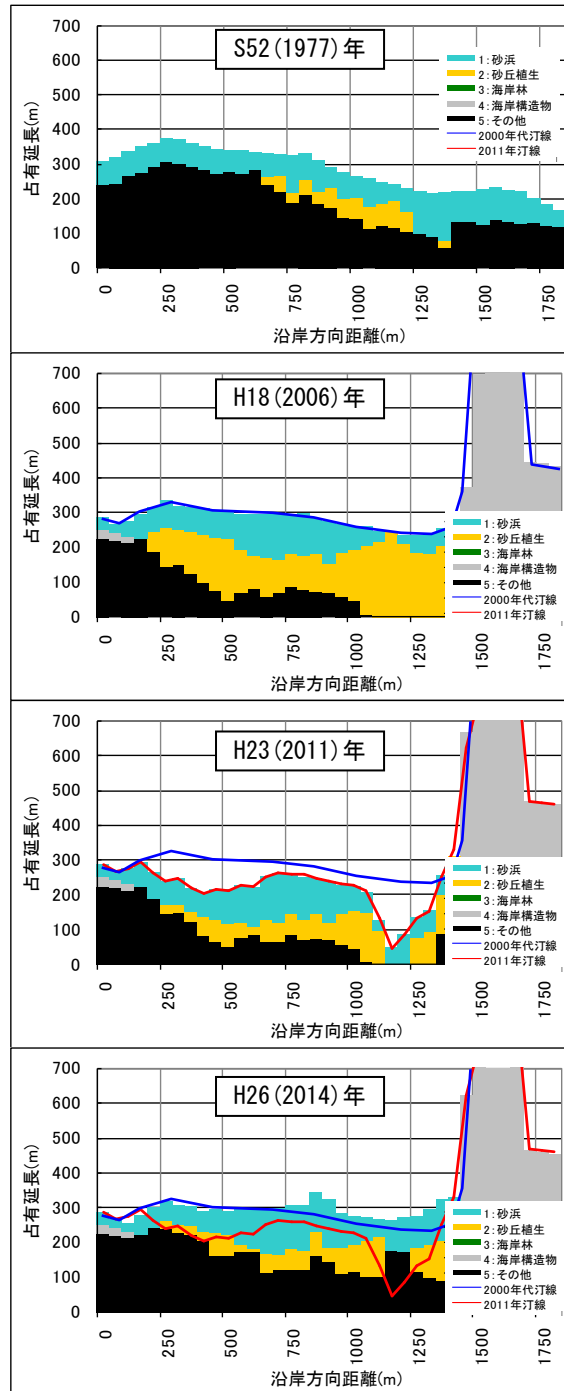
図 2.9 汀線と土地被覆の変化 (久慈市久慈川海岸)
