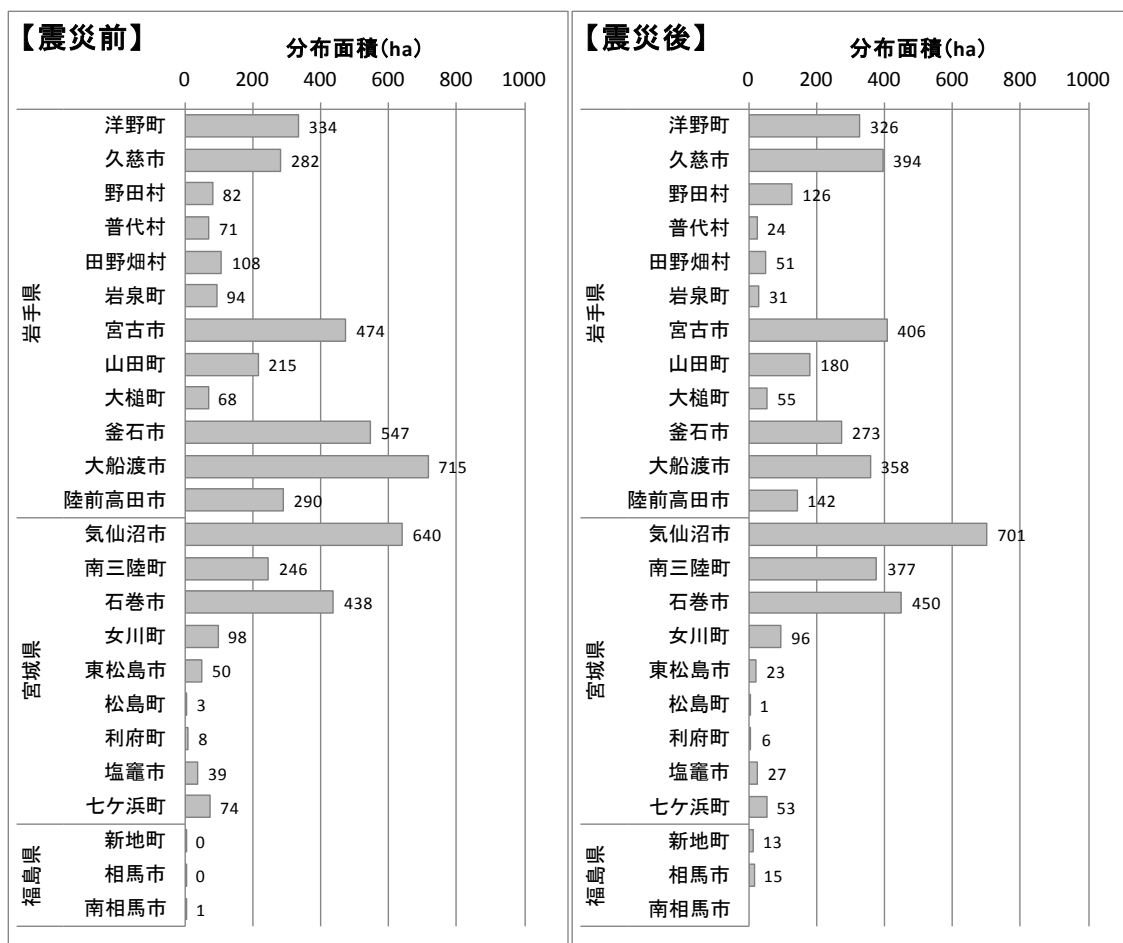
図 2.7 震災前後の大型褐藻類の市町村別分布状況（岩手県～福島県北部）
