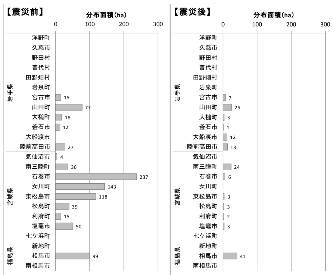
図 2.8 震災前後のアマモ類の市町村別分布状況（岩手県～福島県北部）
