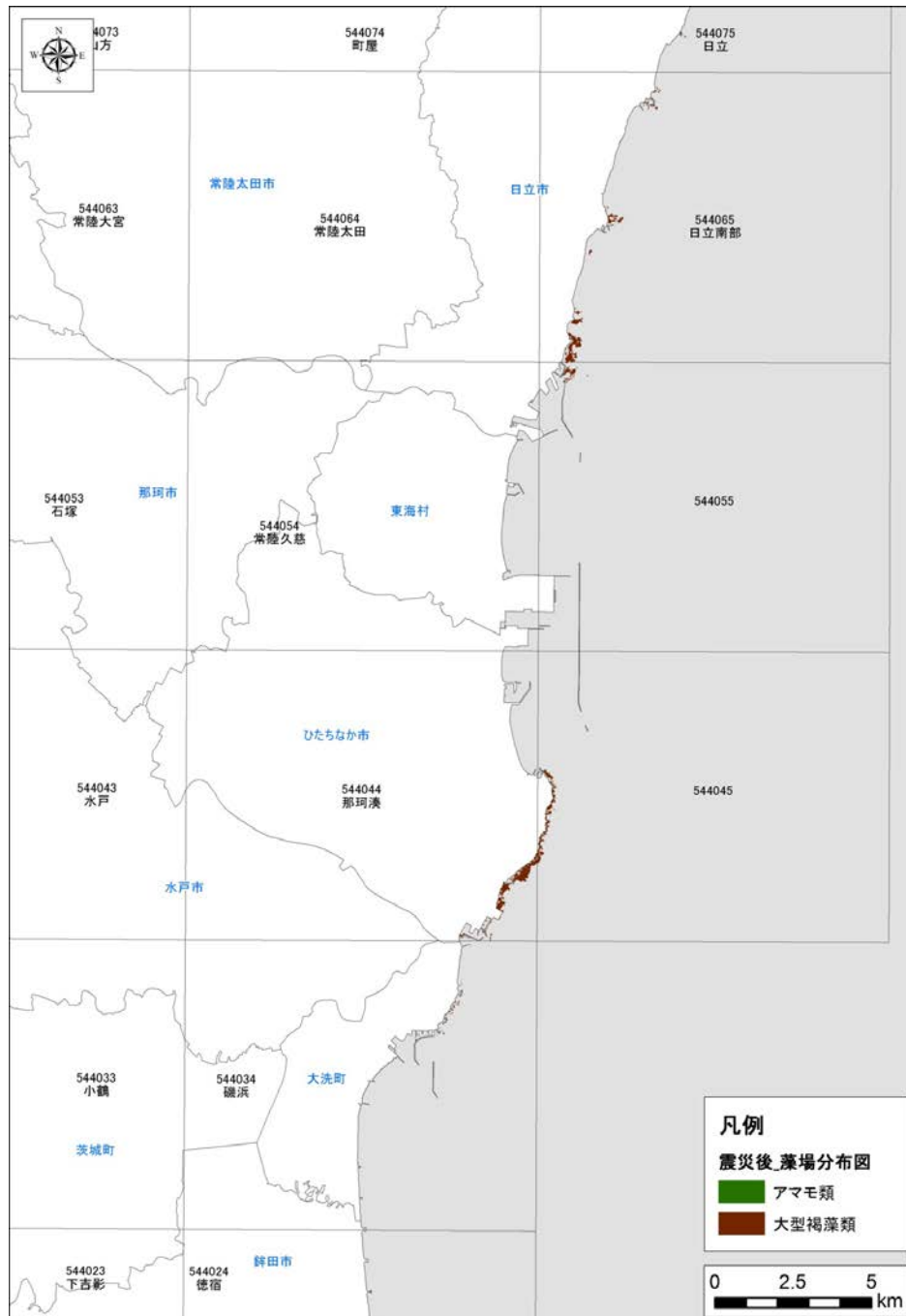
図 2.9 藻場・アマモ場の震災後分布図 (茨城県南部)
