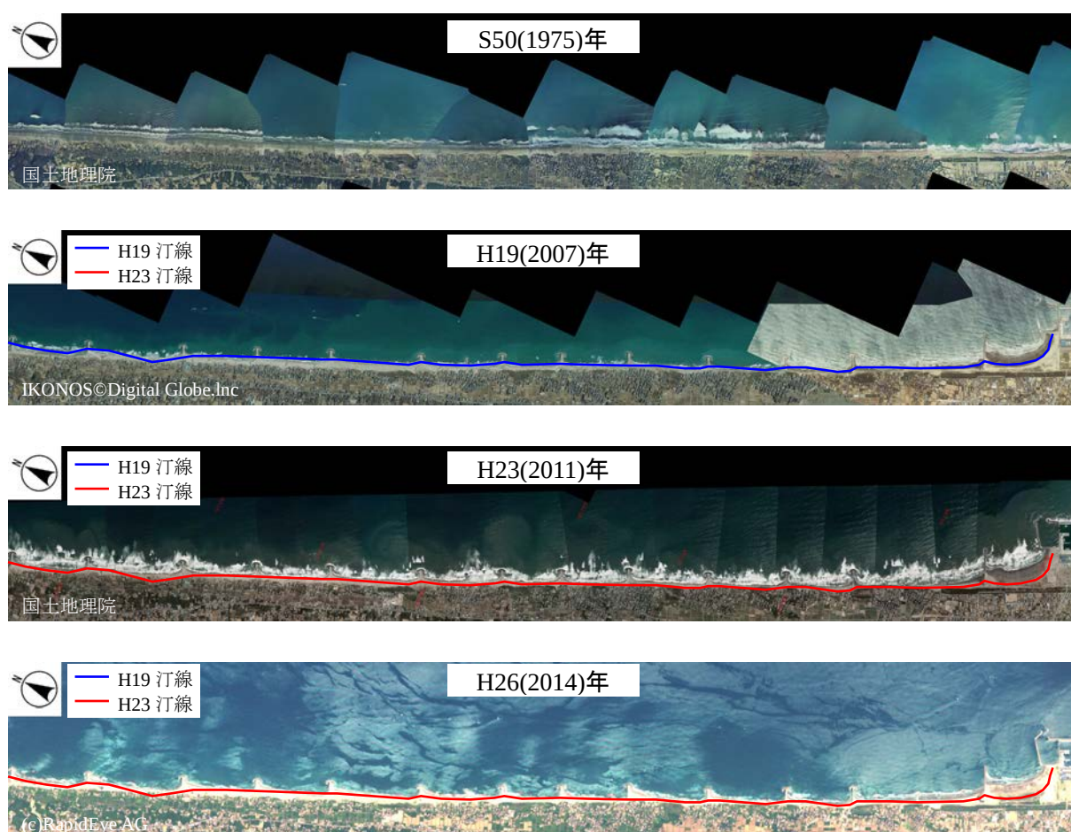
図 2.8 空中写真・衛星画像による海岸の変遷（鹿嶋市鹿島港北海岸）
